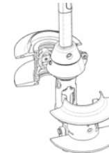
PERFIL DE DOBLE RELINGA + TAMBOR DESMONTABLE, IDEAL PARA REGATAS
